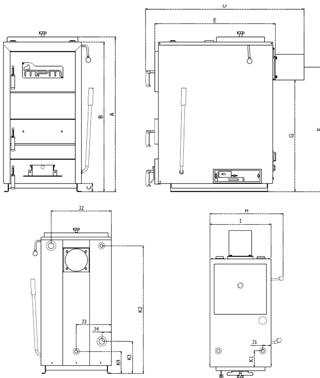
Abbildung 2: Grundlegende Abmessungen des MPM Wood Plus Holzkessels
