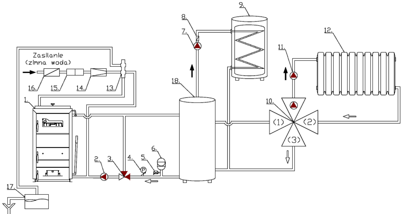
Abbildung 4: Beispielschema für den Anschluss des MPM Wood Plus Holzessels in einem geschlossenen System.
