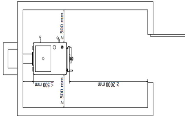
Abbildung 5: Positionierung des Heizkessels im Heizungsraum.
