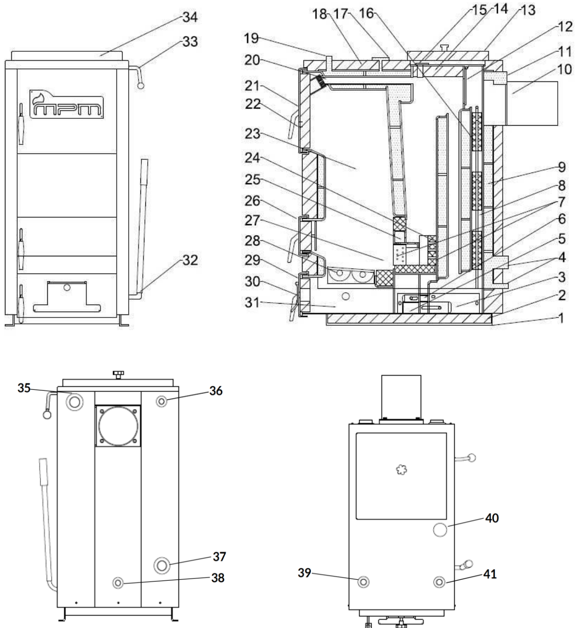
Abbildung 1: Schematische Darstellung eines Seitenladerkessels
